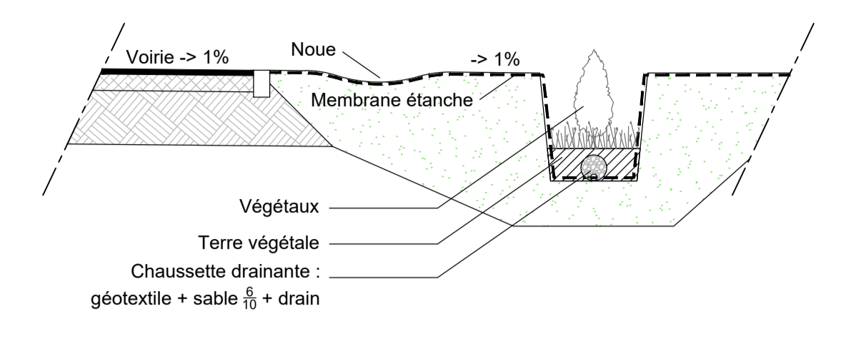
Coupe A-A échelle 1/50 e
